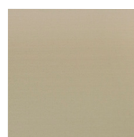
Pumice
